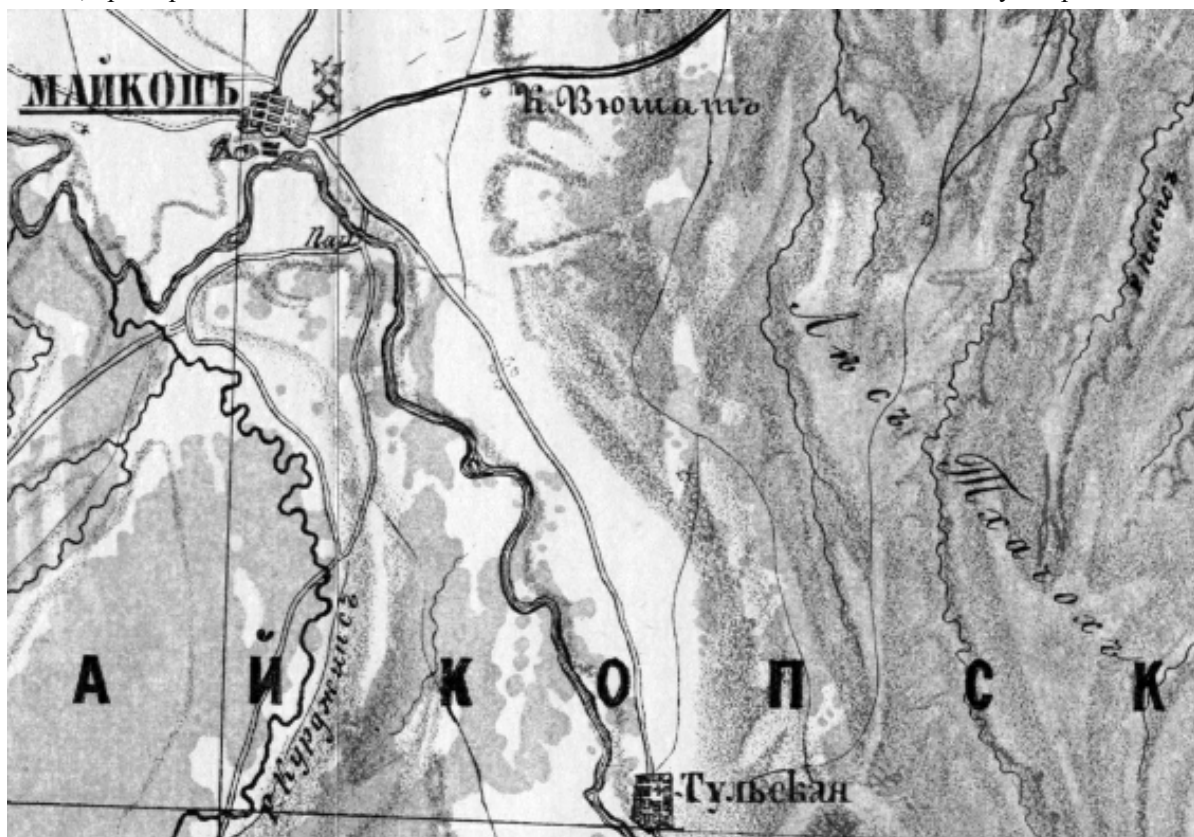
Карта Кубанской области (до 1890 г.) Фрагмент. Курган Вюшат - Ошад, знаменитый Майкопский курган, раскопанный в 1897 г. Название Леса Тхачох следует сопоставить с адыгским понятием тхъачэгъ (тхачег) «название леса, где молились богу». (ТСАЯ. 2006. С. 405). Прим. С.Х.
